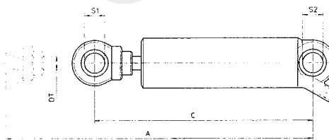
MARTINETTO CON ATTACCHI POSTERIORI
