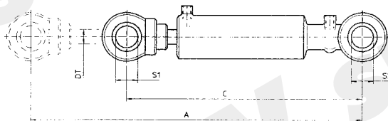
MARTINETTO CON ATTACCHI EQUIDISTANTI
