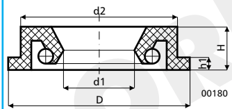
Disegno Drawing 13
