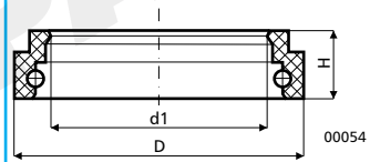
Disegno Drawing 14
