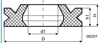
Disegno Drawing 12
