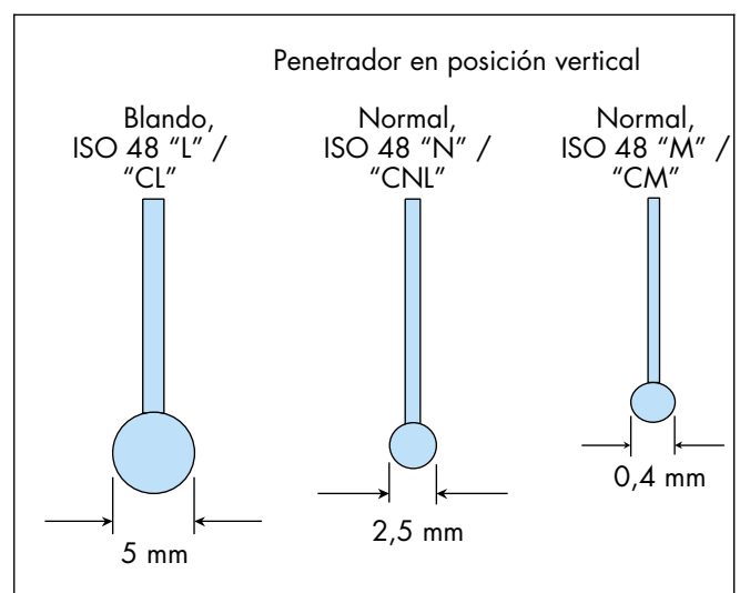
Figura 6 Dimensiones del penetrador, según IRHD
