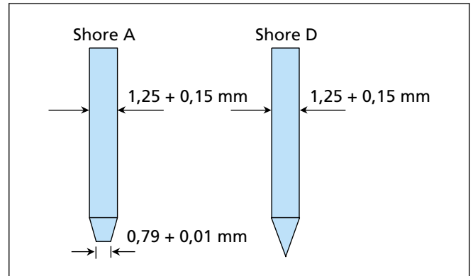
Figura 5 Penetradores de los métodos Shore A y Shore D
