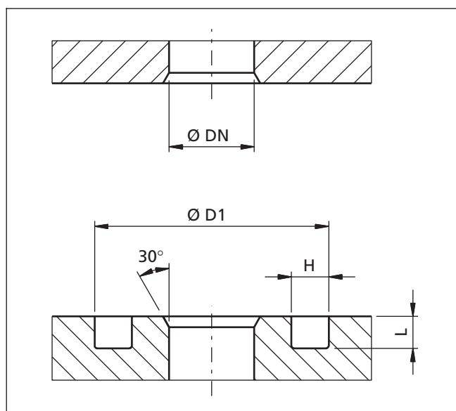
Figura 40 Dimensiones de instalación SAE
