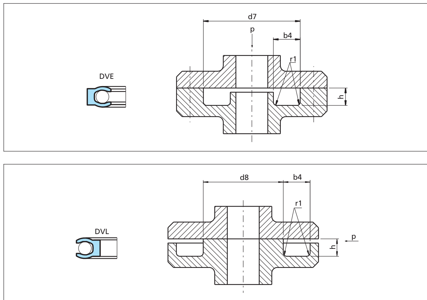
Figura 46 Diagrama de instalación
