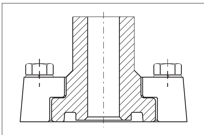
Figura 36 Borda SAE conforme a J518
