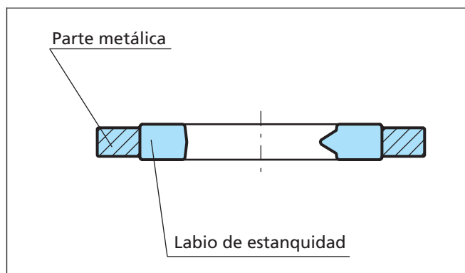
Figura 24 Junta GM2000
