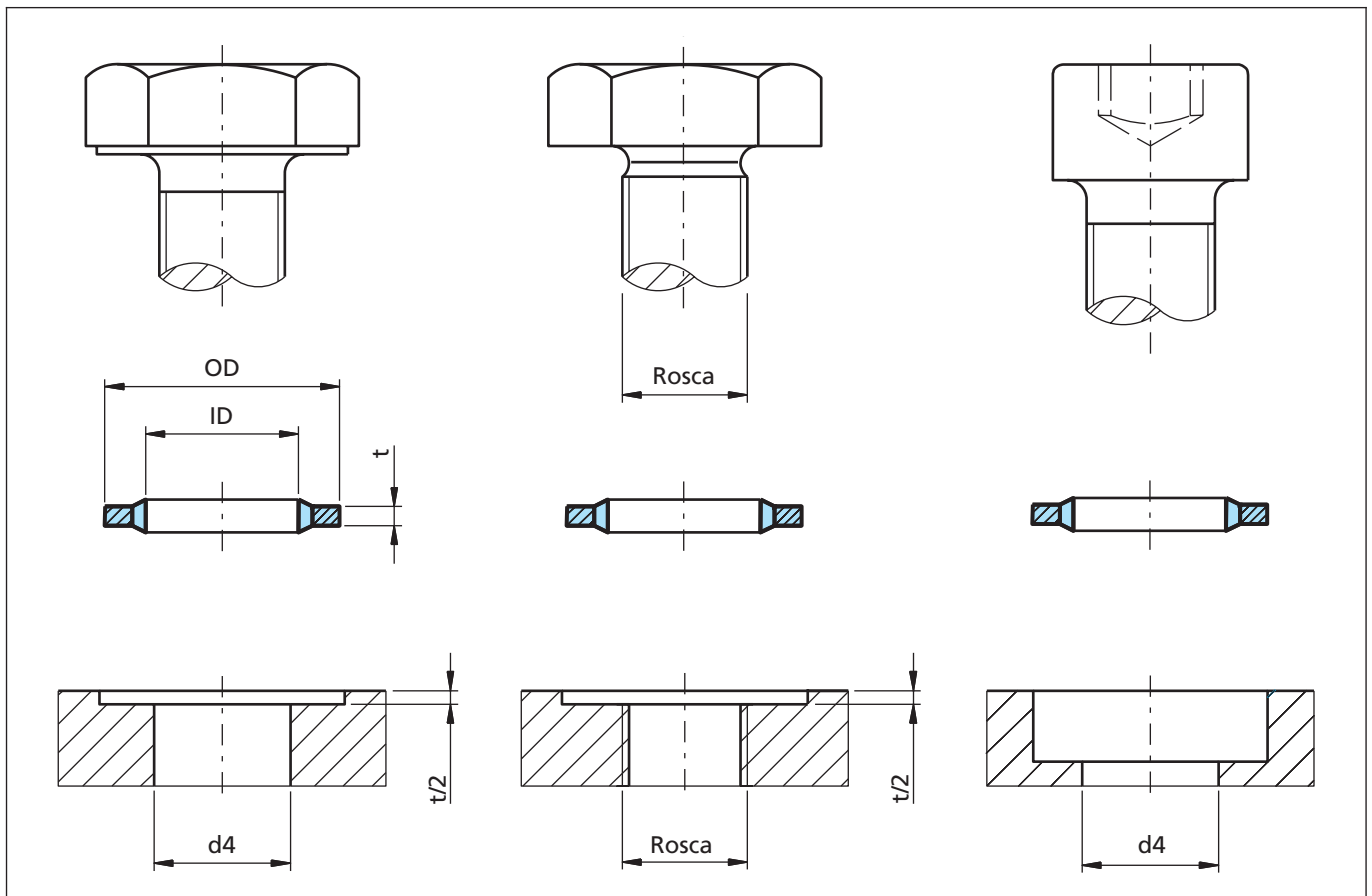
Figura 31 Diagrama de instalación
