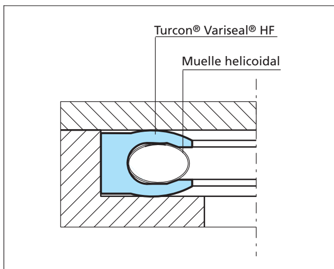
Figura 45 Turcon® Variseal® HF
