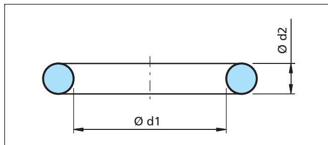
Figura 37 Junta tórica conforme a AS 568 A
