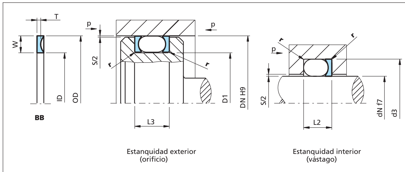
Figura 12 Diagrama de instalación
