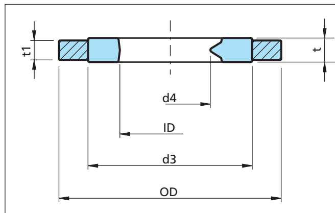
Figura 34 Junta GM2000
